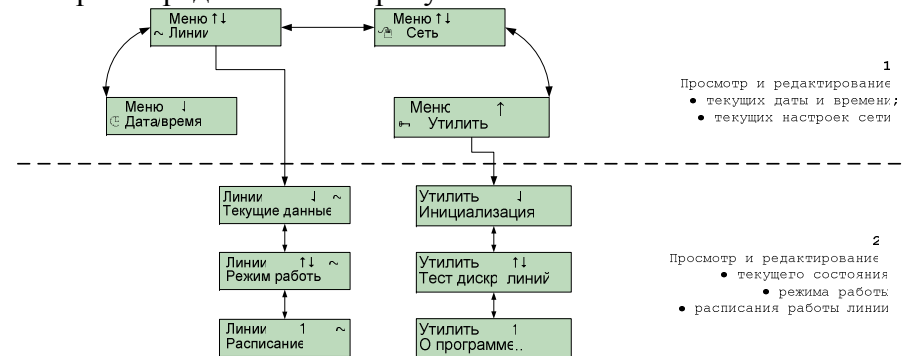
Рисунок 3. Структура меню контроллера «БиКуб-МТ02»
