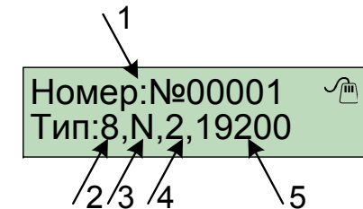
Рисунок 13. Экран конфигурации COM1
