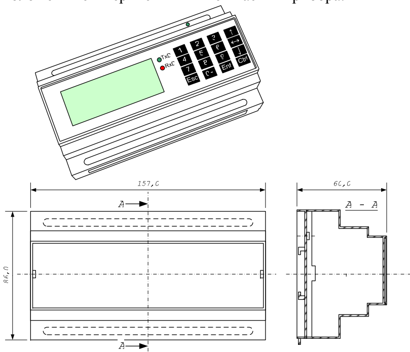
Рисунок 1. Внешний вид контроллера «БиКуб-МТ02».
