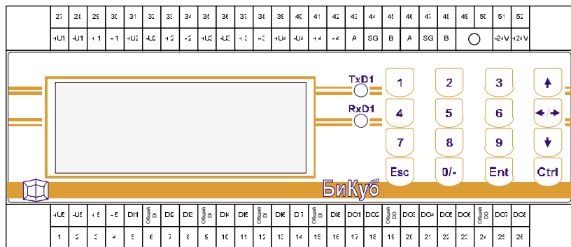
Рисунок 23. Расположение контактов.
