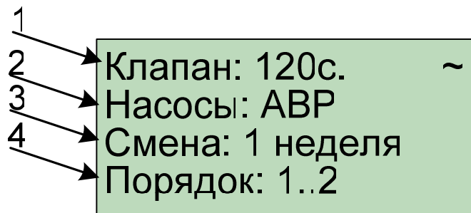
Рисунок 32 . Экран «Оборудование» (экран редактируется)
