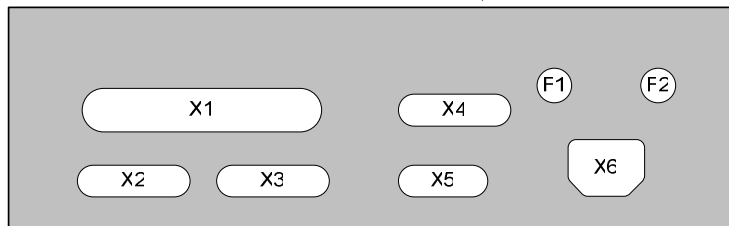
Рисунок 46. Расположение разъемов на нижней панели.
