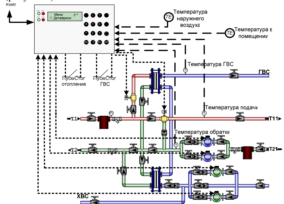
Рисунок 2. Пример применения контроллера «БиКуб-РТ33»
