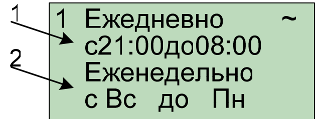
Рисунок 18. Экран расписания режима дежурного отопления (редактируется)
