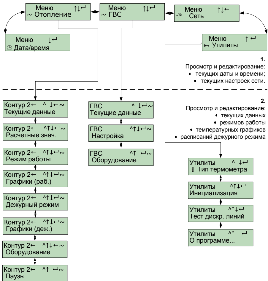
Рисунок 4. Структура меню контроллера «БиКуб-РТ33»
