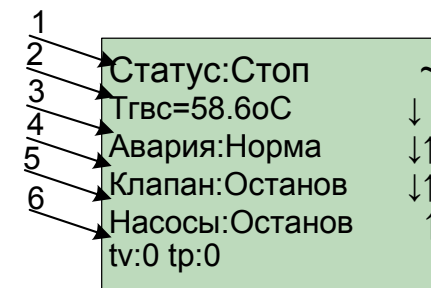
Рисунок 28. Экран текущих данных (экран не редактируется)
