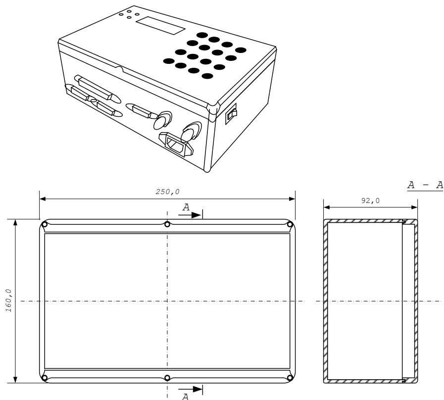
Рисунок 1. Внешний вид контроллера «БиКуб-РТ33»
