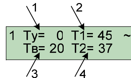
Рисунок 21. Экран «Расчетные значения»
