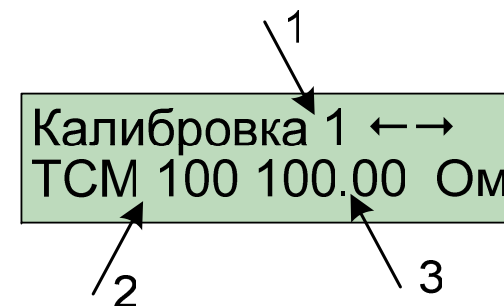
Рисунок 36 Экран «Калибровка» (экран редактируется)
